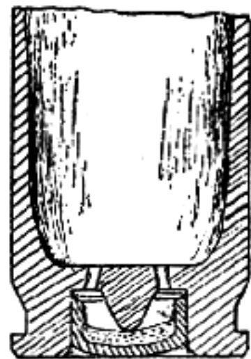
SEPARATE ANVIL PRIMER
