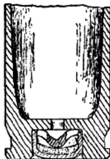
SEPARATE ANVIL PRIMER
